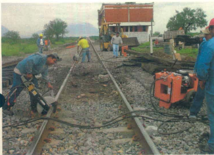
Maquina Hidráulica (Incluye los siguientes accesorios: Apriete de fijaciones, cortar riel, esmerilar, cortamazarota, taladrar, Mod. 2007
